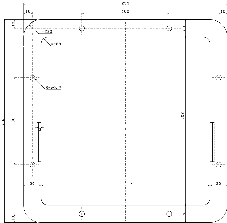
埋め込みキット™ FR-26 材質 SUS 厚さ 1.5mm 表面処理：塗装グレー
