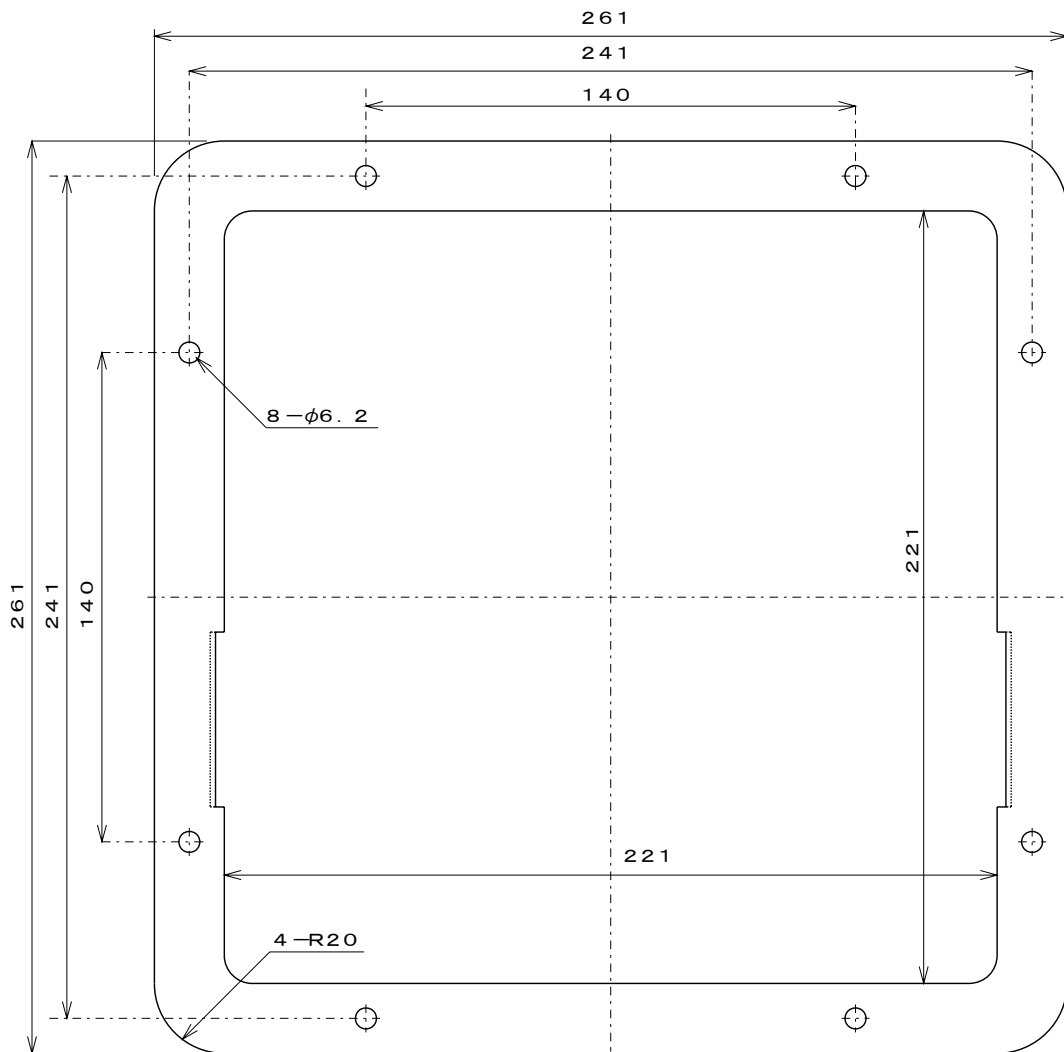
埋込みキッド FR-28 材質: SUS t = 1.5 mm 表面処理: 塗装グレー
